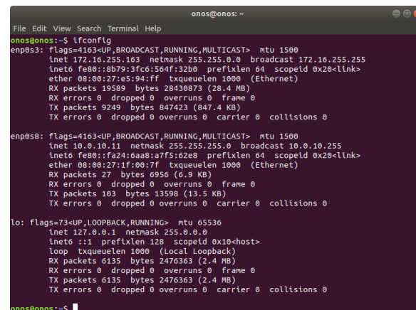
Εικόνα 21: Ρυθμίσεις κάρτας δικτύου - ONOS Controller VM
