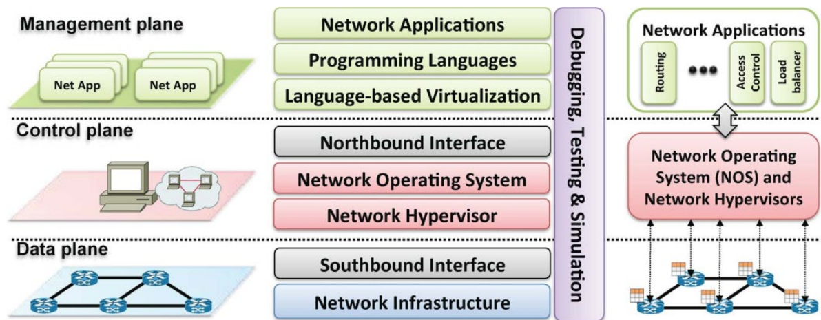
Εικόνα 7: Επίπεδα αρχιτεκτονικής SDN (Πηγή: (Kreutz et al., 2015))
